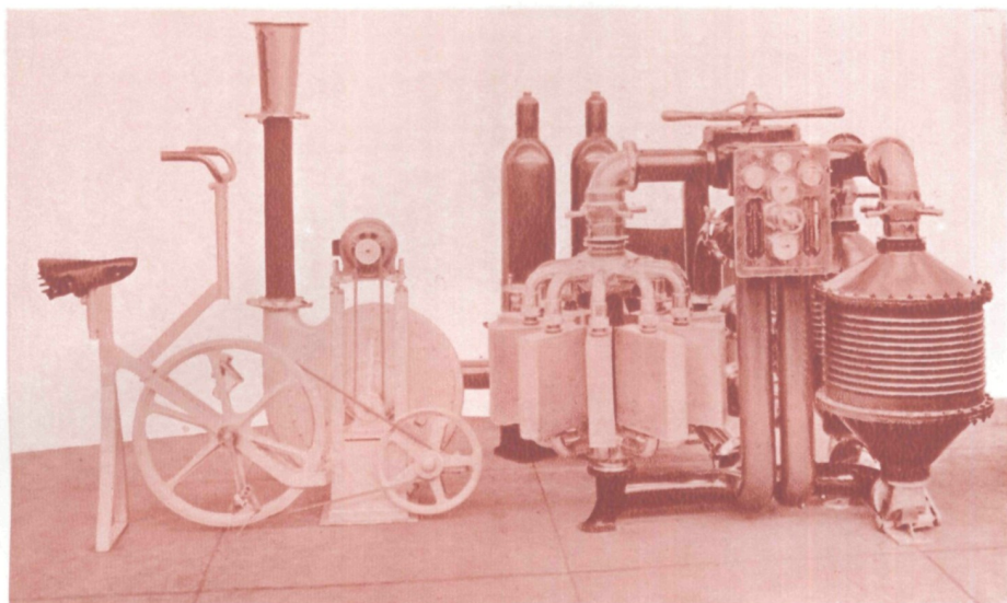
Ensemble de protection contre tous les gaz de combat Système "S. I. C. A. A." (Breveté dans tous les pays)
