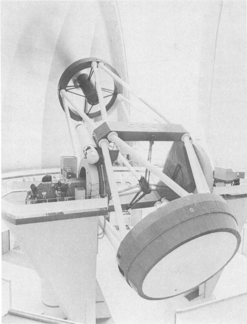
The 6m Telescope (BTA)
