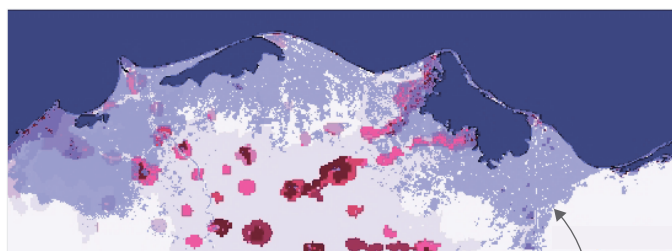
(d) 2100, at 1.7 m sea level rise (SSP5-high-end)
